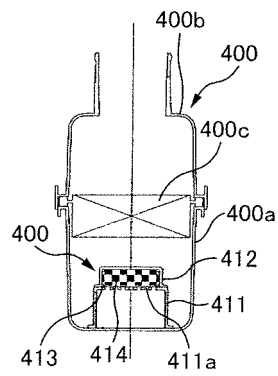
sec D-D FIG. 9C
