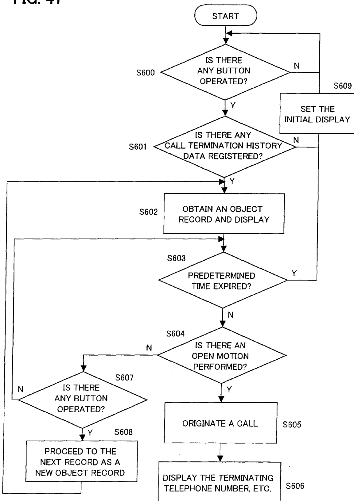
FIG. 41
