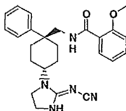
trans-N-[4-(2-Cyanoimino-imidazolin-1-yl)-1-phenyl-cyclohexylmethyl]-2-methoxybenzamide
