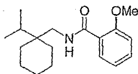
N-(1-Isopropyl-cyclohexylmethyl)-2-methoxy-benzamide
