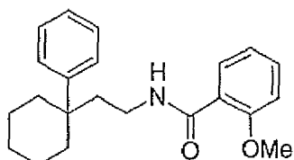
2-Methoxy-N-[2-(1-phenyl-cyclohexyl)-ethyl]-benzamide
