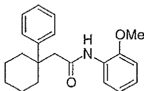
N-(2-Methoxy-phenyl)-2-(1-phenyl-cyclohexyl)-acetamide
