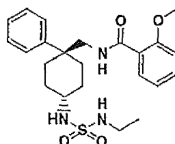
trans-2-Methoxy-N-[4-(N-ethyl-N'-sulfenylureido)-1-phenylcyclohexylmethyl]-benzamide
