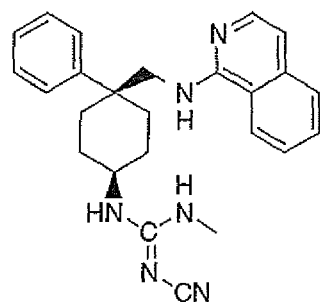
Ex. 411
