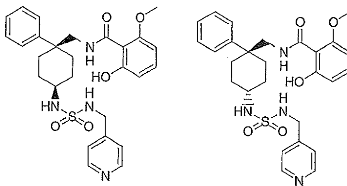
Ex. 572
