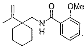
N-(1-Isopropenyl-cyclohexylmethyl)-2-methoxy-benzamide
