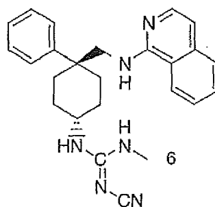
Ex. 412
