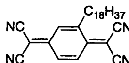
C 18 TCNQ
