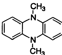
(Me) 2 P
