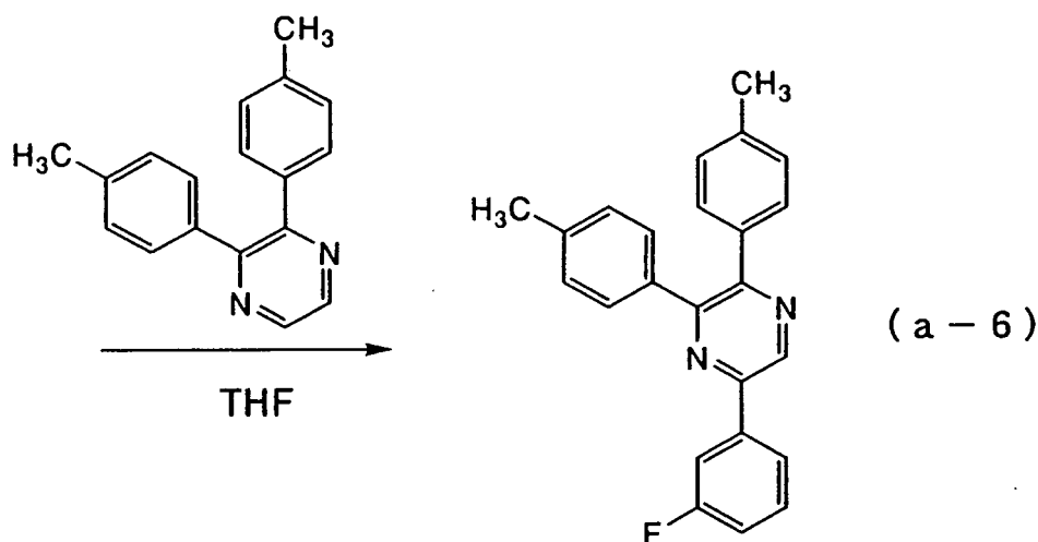
HMdppr-3FP
