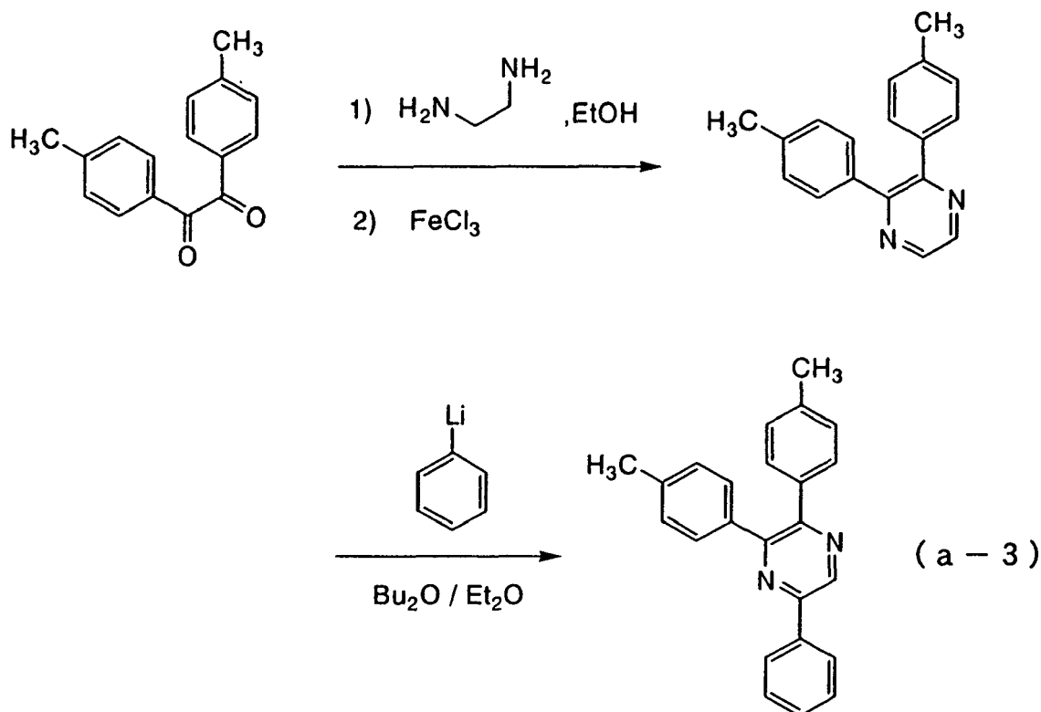
HMdppr-P
