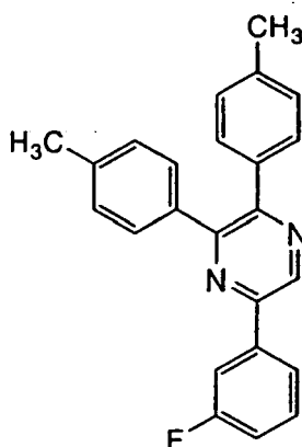
HMdppr-3FP
