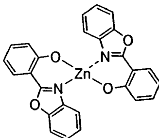
\text{Zn(PBO)}_2
