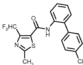
(6-29) N -(4'-Brom-1,1'-biphenyl-2-yl)-4-(difluormethyl)-2-methyl-1,3-thiazol-5-carboxamid (bekannt aus WO 03/066610) der Formel
