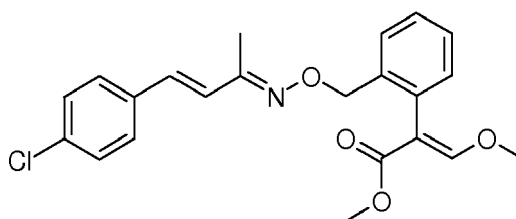
(2-15) Enestrobin (bekannt aus EP-A 0 936 213) der Formel
