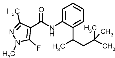
(6-9) 3-(Difluormethyl)-1-methyl-N-[2-(1,3,3-trimethylbutyl)phenyl]-1H-pyrazol-4-carboxamid der Formel
