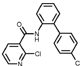
(6-19) Furametpyr (bekannt aus EP-A 0 315 502) der Formel
