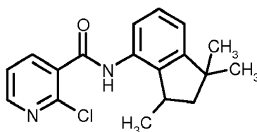
(6-18) Boscalid (bekannt aus DE-A 195 31 813) der Formel
