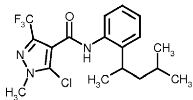
(6-7) 1,3-Dimethyl-N-[2-(1,3,3-trimethylbutyl)phenyl]-1H-pyrazol-4-carboxamid der Formel
