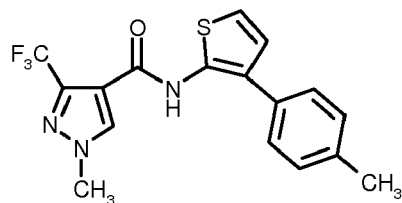
(6-21) Penthiopyrad (bekannt aus EP-A 0 737 682) der Formel
