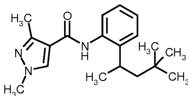
(6-7) 1,3-Dimethyl-N-[2-(1,3,3-trimethylbutyl)phenyl]-1H-pyrazol-4-carboxamid der Formel
