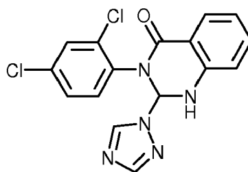
(3-26) Amisulbrom (bekannt aus JP-A 2001-187786) der Formel
