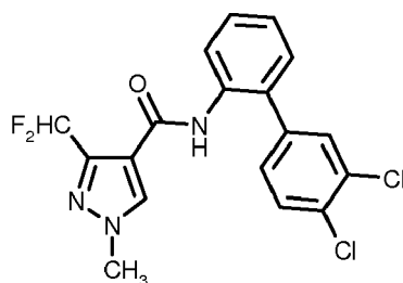
(6-52) N-(3',4'-Dichlor-5-fluor-1,1'-biphenyl-2-yl)-3-(difluormethyl)-1-methyl-1H-pyrazol-4-carboxamid (bekannt aus WO 2005/123689) der Formel
