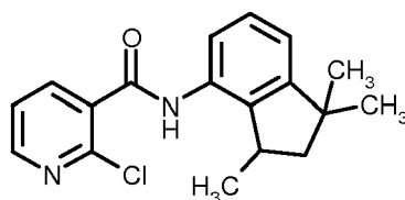
(6-18) Boscalid (bekannt aus DE-A 195 31 813) der Formel
