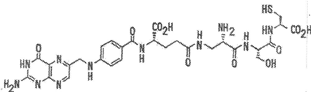
EC13 (Pte-L-γGlu-L-βDpr-L-Ser-L-Cys)
