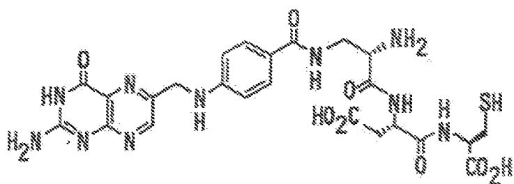
EC31 (Pte-L-βDpr-L-Asp-L-Cys)
