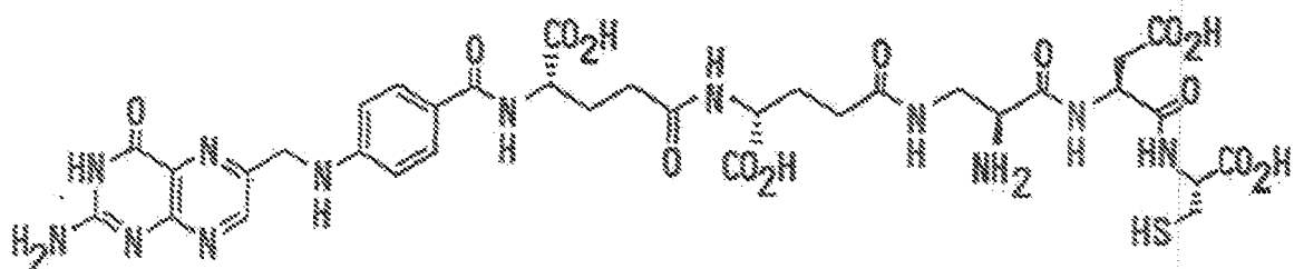
EC14 (Pte-L-γGlu-D-γGlu-L-βDpr-L-Asp-L-Cys)
