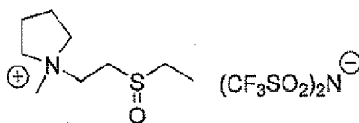
Sulfoxide IL 5
