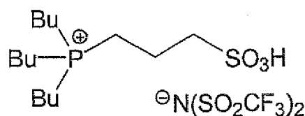
IL3
