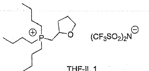
THF-IL 1
