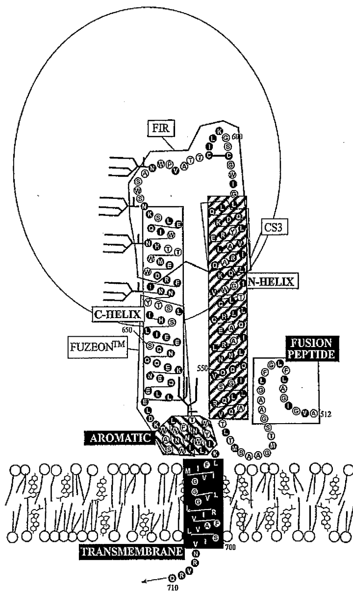
HIV-1 TM Figure 7
