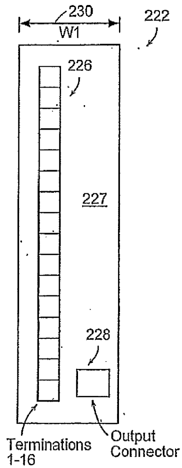
16 Output Module
