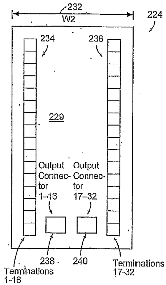
32 Output Module
