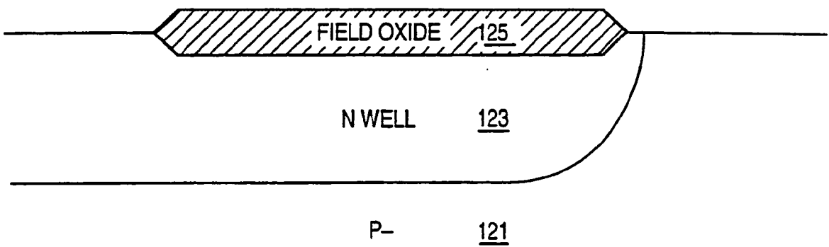
FIG. 11b
