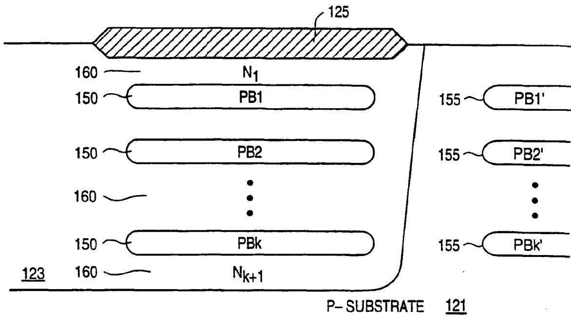
FIG. 11e
