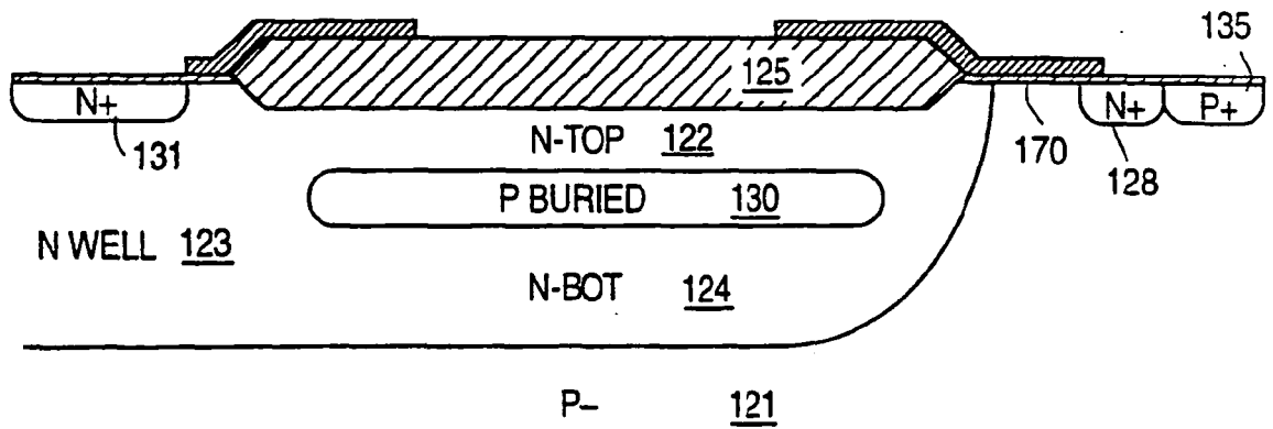
FIG. 11h
