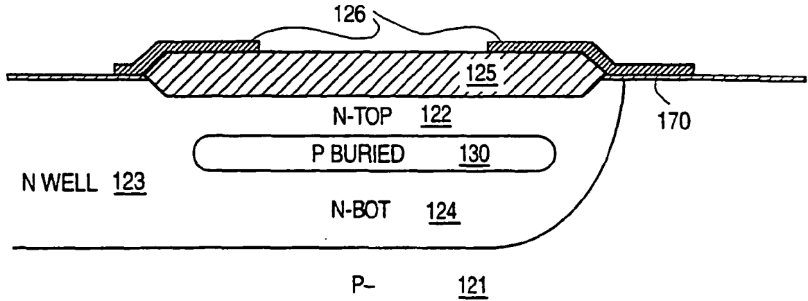
FIG. 11g
