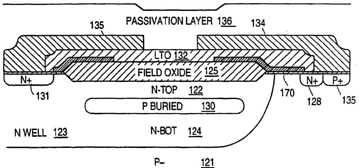
FIG. 11i
