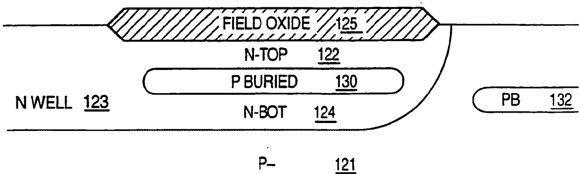
FIG. 11c
