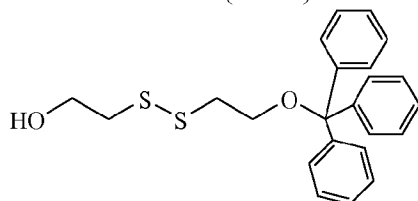
2-((2-(Trityloxy)ethyl)disulfanyl)ethanol ( LI-1c )
