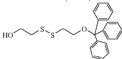
2-((2-(Trityloxy)ethyl)disulfanyl)ethanol ( LI-1c )
