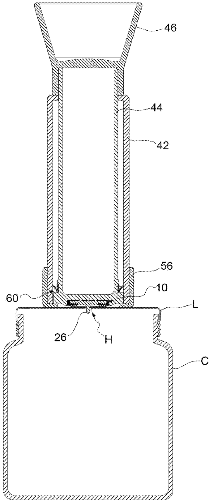
FIG.3f
