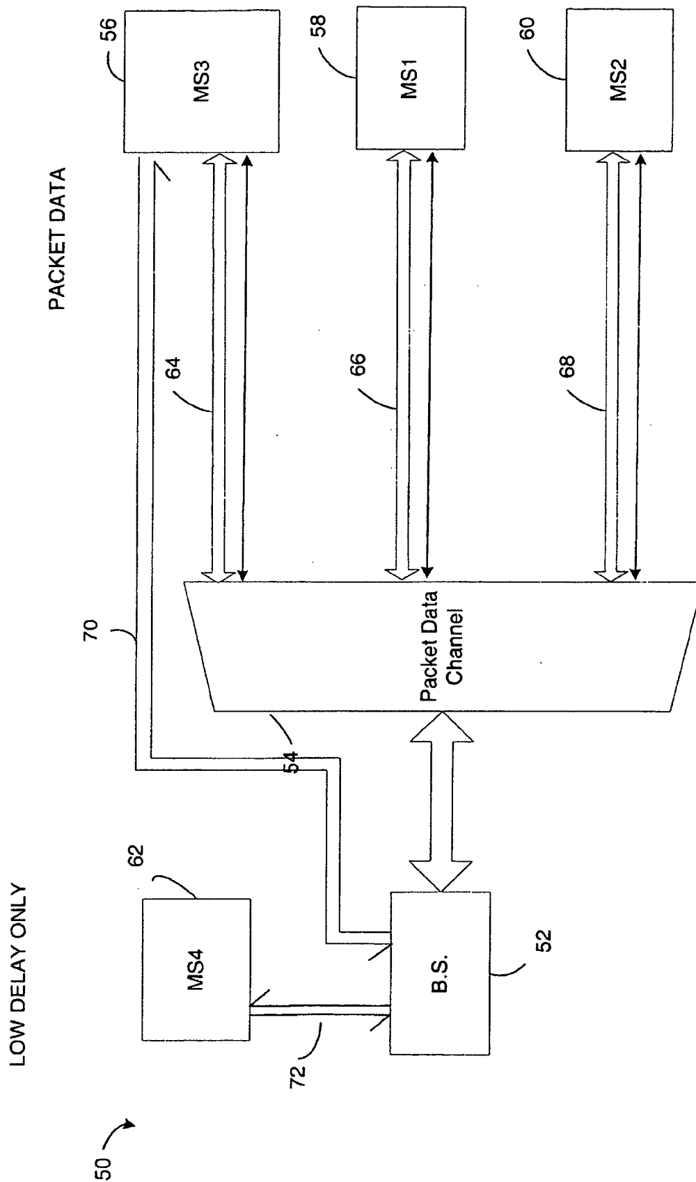
FIG. 5 DRC
