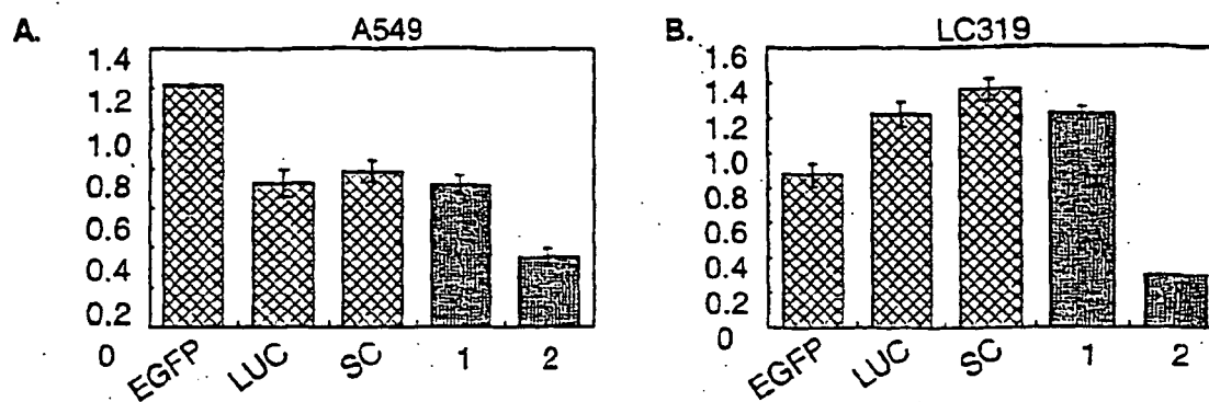
Fig. 3-3 1191: COX17
