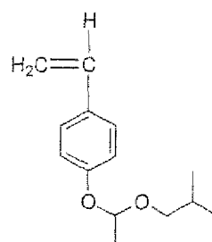
Monomer (4)
