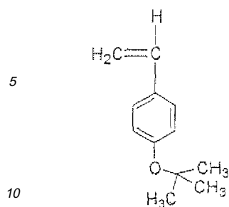
Monomer (1)
