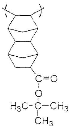
( B-25 )
