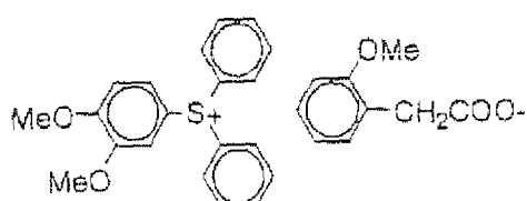
(II-29)
