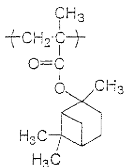
(B-14)
