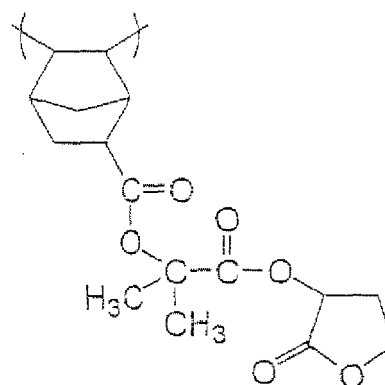
( B-24 )
