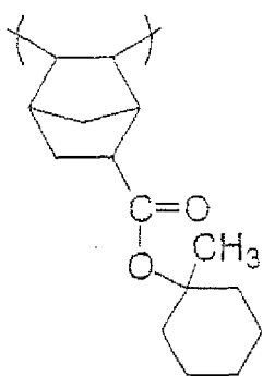
( B-22 )
