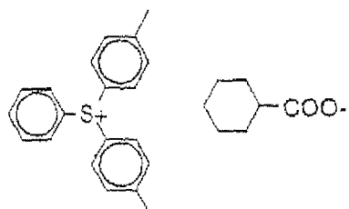
(II-22)
