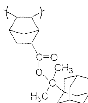
(B-21)
