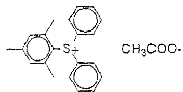
(II-28)
