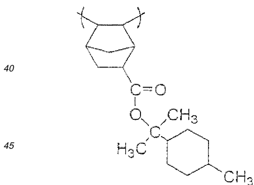
(B-19)
