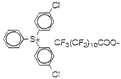
(II-54 f)
