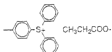
(II-31)
