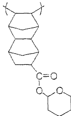
( B-26 )
