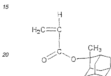
Monomer (3)
