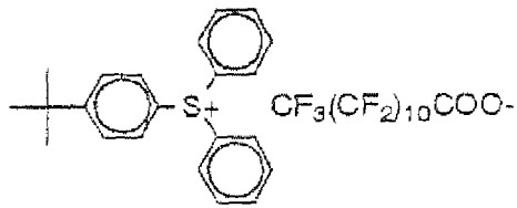
(II-53 f)
