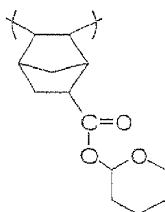
(B-17)
