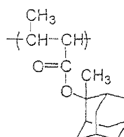
(B-9)
