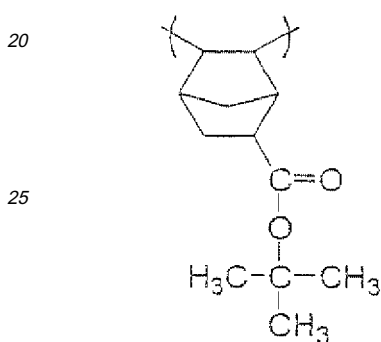
(B-16)
