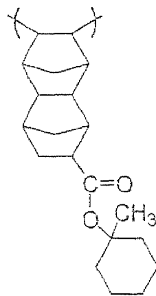
(B-30)
