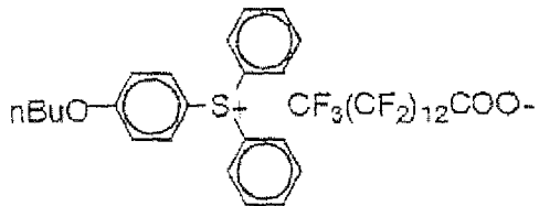
(II-57 f)
