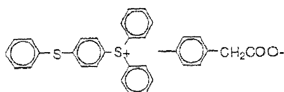
(II-23)
