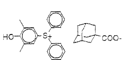
(II-21)
