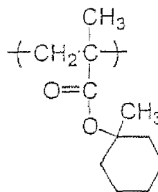
(B-6)
