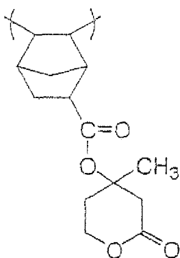
( B-23 )
