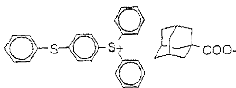
(II-25)
