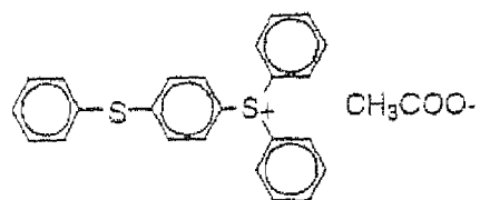
(II-24)
