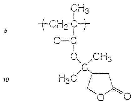
(B-13)
