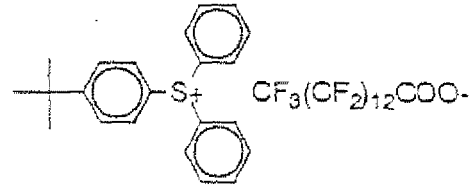
(II-58 f)
