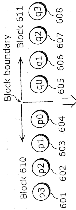
Fig. 9A Before filtering
