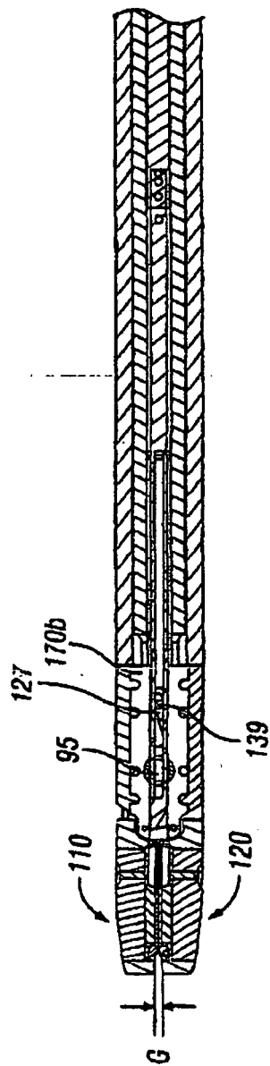
FIG. 8C
