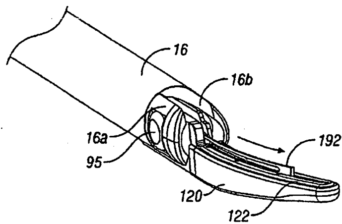
FIG. 10D
