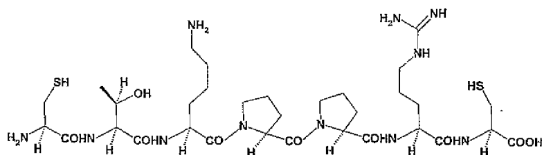
H-Cys-Thr-Lys-Pro-Pro-Arg-Cys-OH (CTKPPRC)
