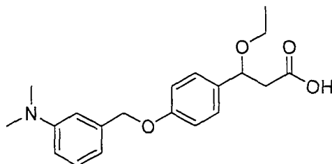
(8A) Ethyl 3-(4-((3-(dimethylamino)benzyl)oxy)phenyl) -3-ethoxypropionate
