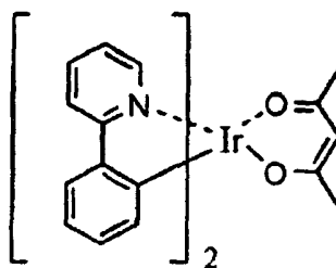
Ir(ppy) 2 (acac)
