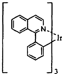
Ir(plq) 3
