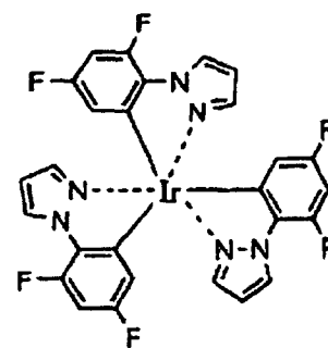
Ir(dfppz) 3
