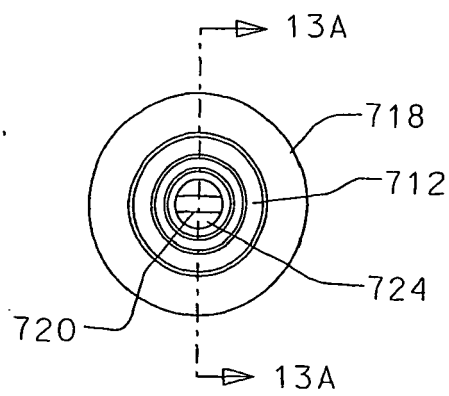
FIG. 13C
