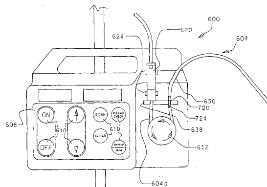
FIG. 13E
