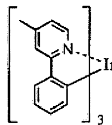
\text{Ir(mpyp)}_3
