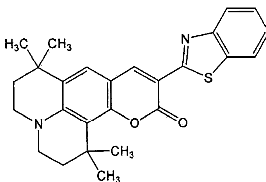
C545T
