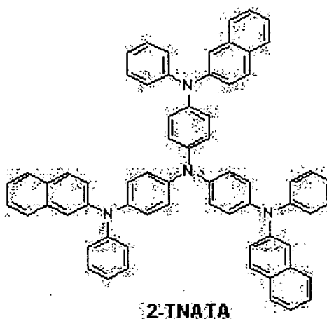
m-MTDATA
