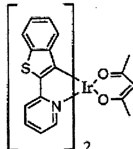
Btp 2 Ir(acac)
