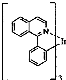
Ir(plq) 3
