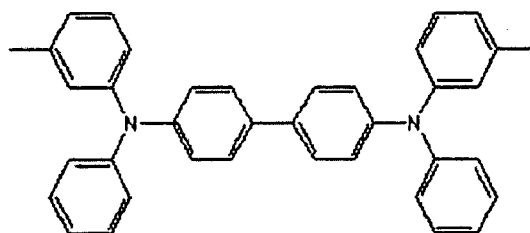
TPD
