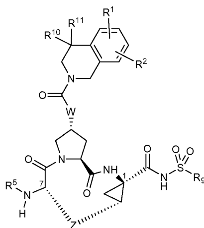
(VIIIa)
