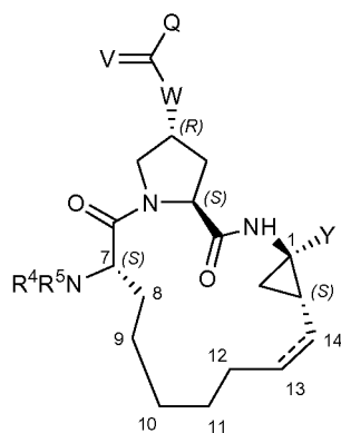
(VIIa)
