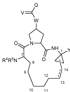
(VII)
