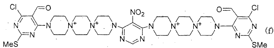
[Chem. 25]
