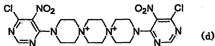
[Chem. 6]
