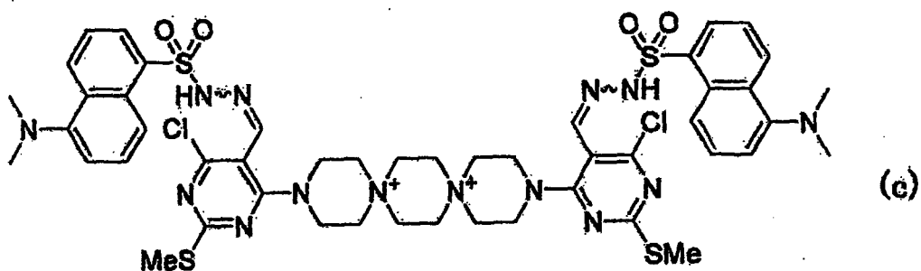
[Chem. 5]
