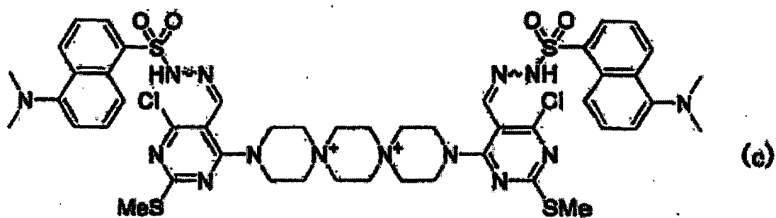
[Chem. 5]
