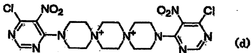
[Chem. 6]
