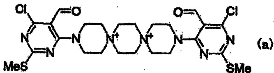
[Chem. 3]
