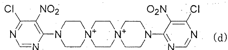
[Chem. 23]
