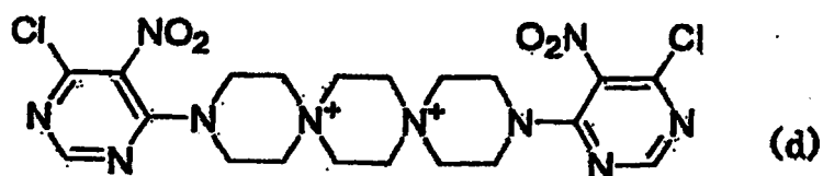
[Chem. 6]
