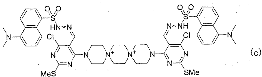
[Chem. 5]
