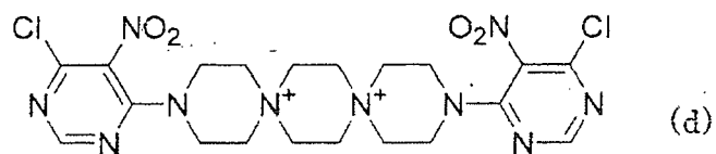
[Chem. 6]
