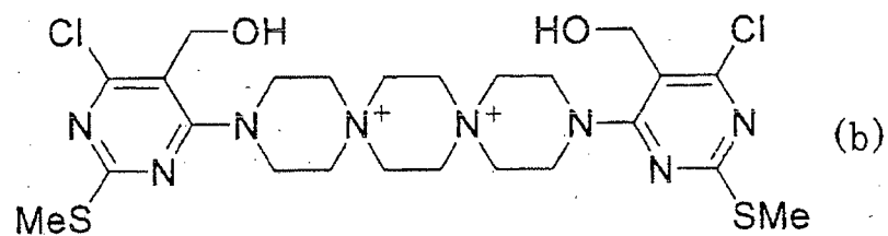
[Chem. 5]
