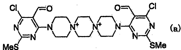
30 [Chem. 3]
