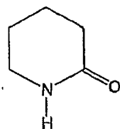
caprolactam
