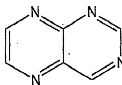
pteridine
