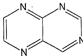
pteridine
