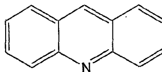
acridine
