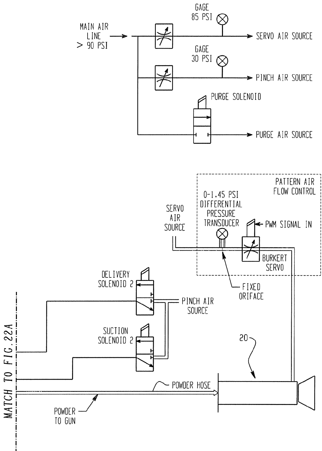
Fig. 22B
