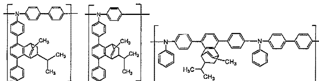
[Chem. 6]
