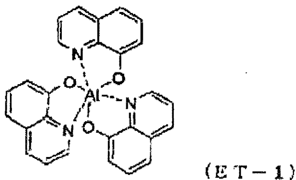
[Chem. 65]
