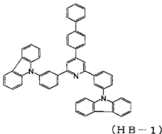
[Chem. 64]
