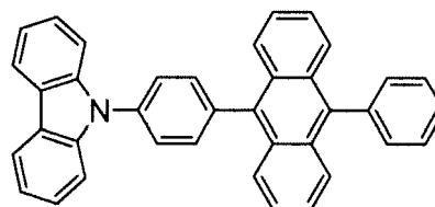
CzPA
