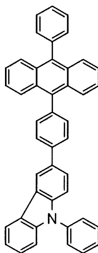
PCzPA
