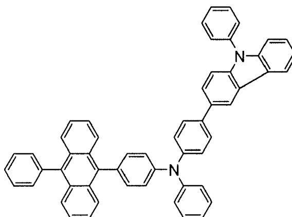
PCBAPA
