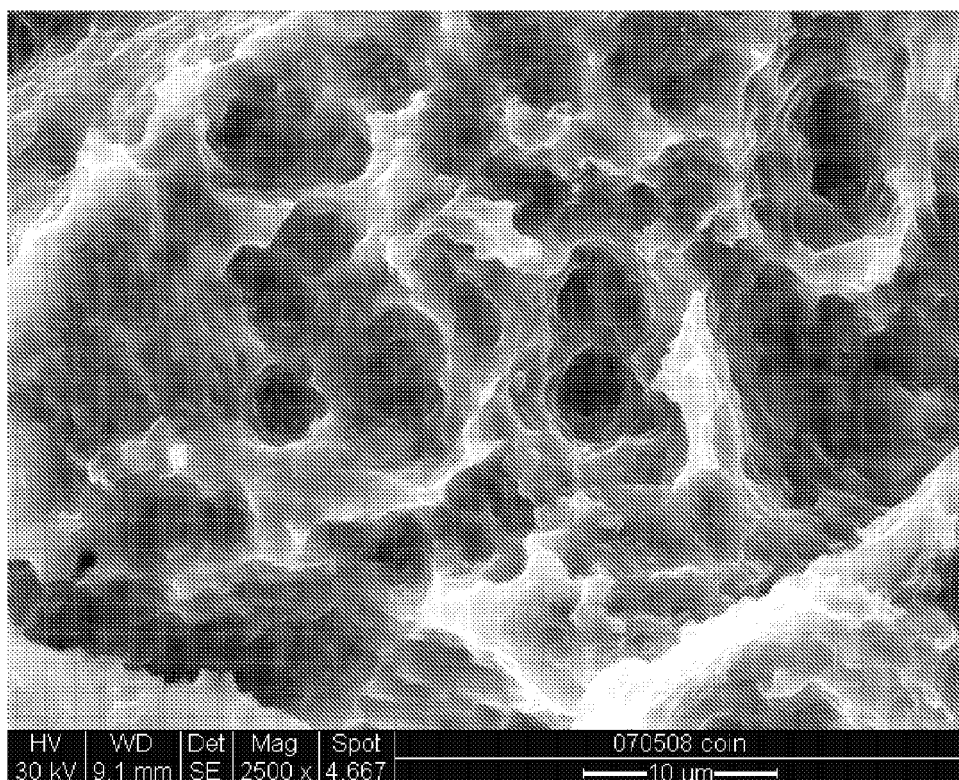
Fig. 12c
