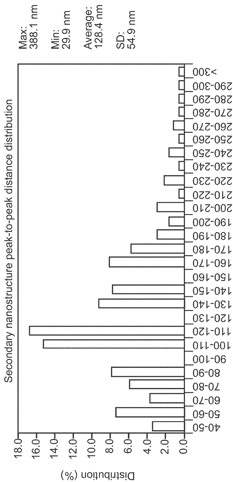
Fig. 17c
