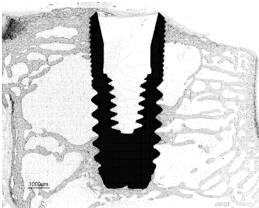
Fig. 23a
