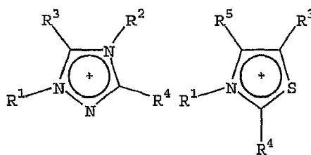
1,2,4-TRIAZOLIUM
