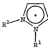
PYRAZOLIUM
