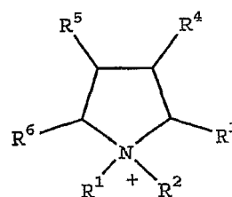
PYRROLIDIUM
