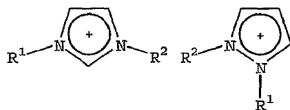
IMIDAZOLIUM
