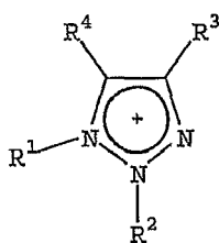
1,2,3-TRIAZOLIUM
