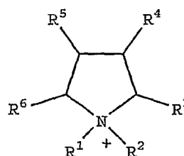
PYRROLIDIUM
