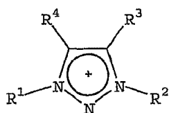
1,2,3-TRIAZOLIUM
