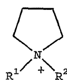
PYRROLIDIUM
