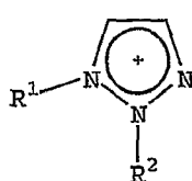
1,2,3-TRIAZOLIUM
