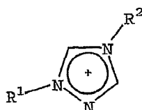
1,2,4-TRIAZOLIUM
