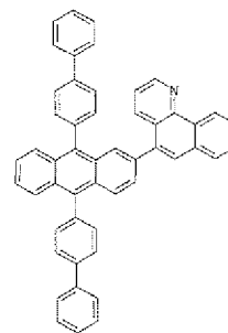
[Formula 1-44]
