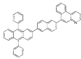
[Formula 3-28]
