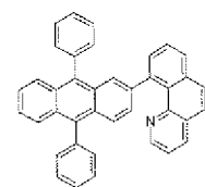
[Formula 1-85]
