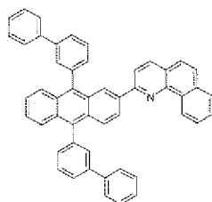
[Formula 1-18]
