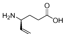
Vigabatrin-(b)
