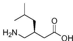
Pregabalin-(d)
