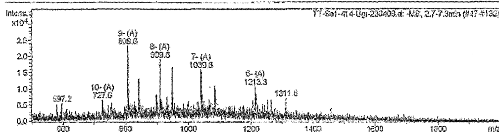
-MS, 2.7-7.3min (#47-#132)
