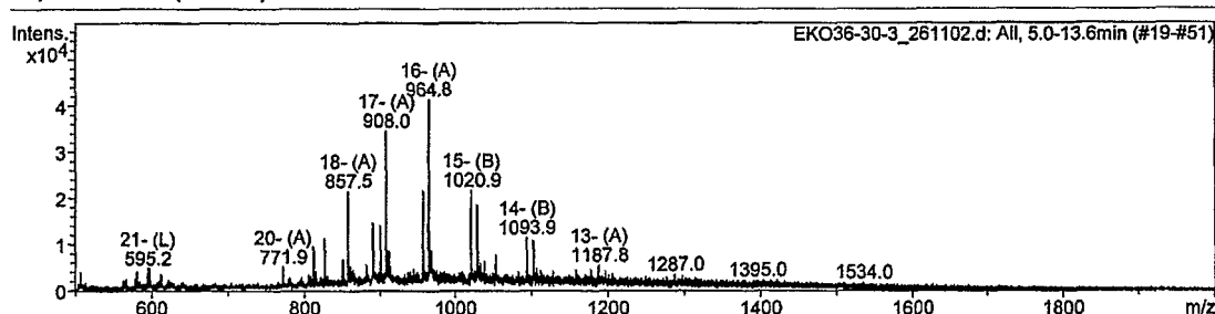
All, 5.0-13.6min (#19-#51)
