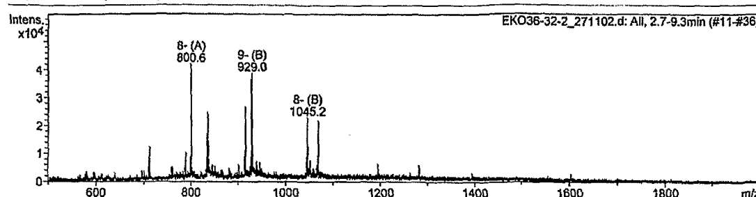
All, 2.7-9.3min (#11-#36)
