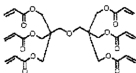
Monomer A
