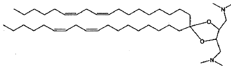
DLin-K 2 -DMA or
