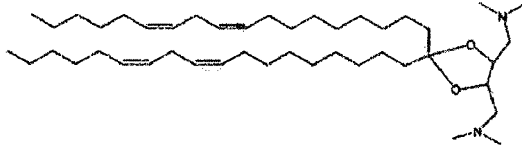
DLin-K 2 -DMA oder
