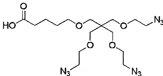
5-(3-(2-azidoethoxy)-2,2-bis((2-azidoethoxy)methyl)propoxy)pentanoic acid
