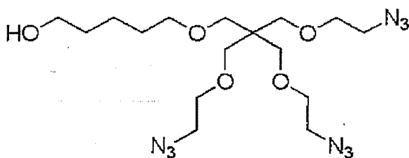
5-(3-(2-azidoethoxy)-2,2-bis((2-azidoethoxy)methyl)propoxy)pentan-1-ol
