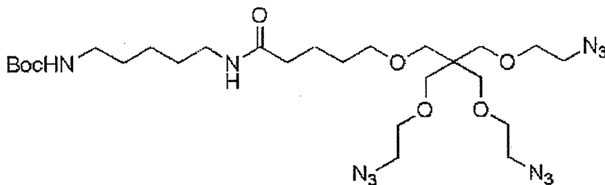
Tert-butyl 5-(5-(3-(2-azidoethoxy)-2,2-bis((2-azidoethoxy)methyl)propoxy)pentanamido)pentylcarbamate
