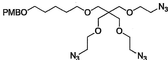
1-((5-(3-(2-azidoethoxy)-2,2-bis((2-azidoethoxy)methyl)propoxy)pentyl)oxy)methyl)-4-methoxybenzene
