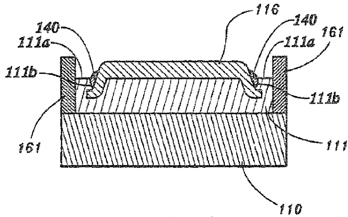
FIG. 5G
