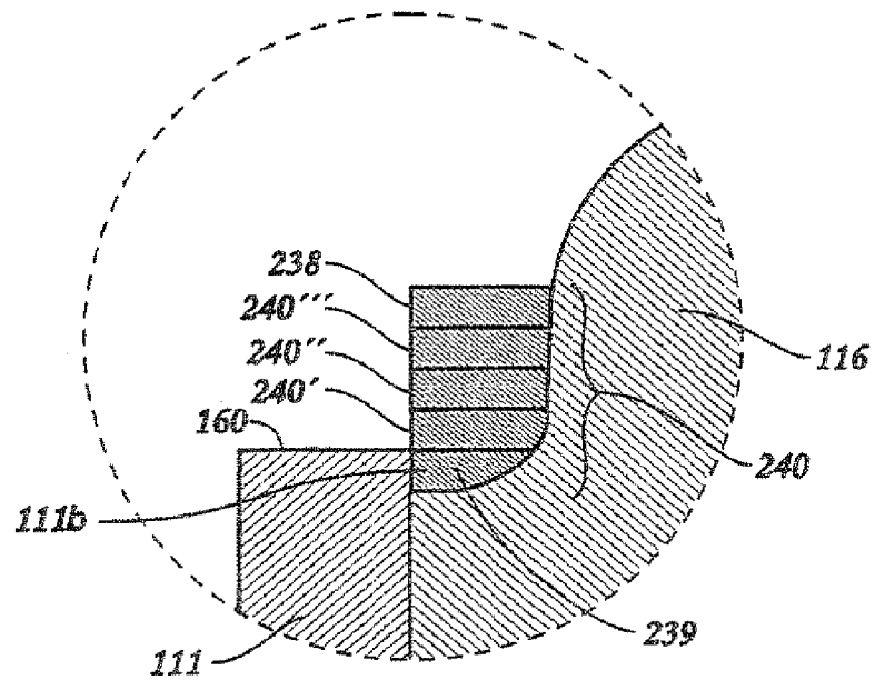
FIG. 5F
