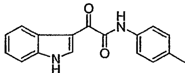
95) 2-indol-3-yl-2-oxo-N-p-tolyl-acetamide
