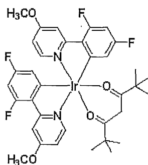
(F_2ppy)_2Ir(tmd)
