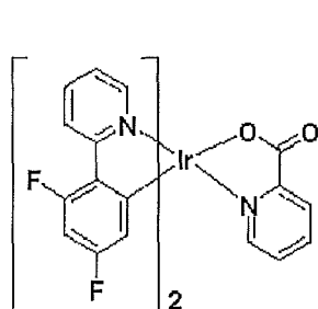
F_2Irpic
