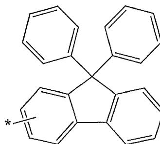
Formula 5E
