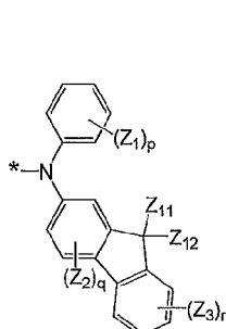
Formula 6G
