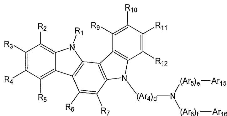
Formula 3e
