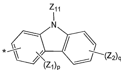
Formula 4E
