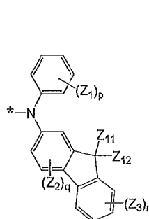
Formula 6G
