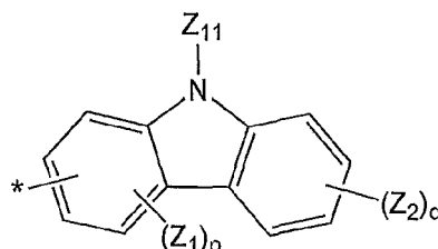
Formula 4E
