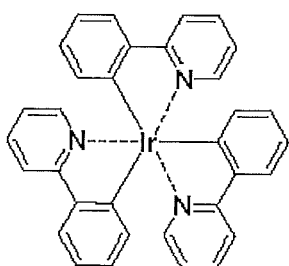
Ir(ppy) 3
