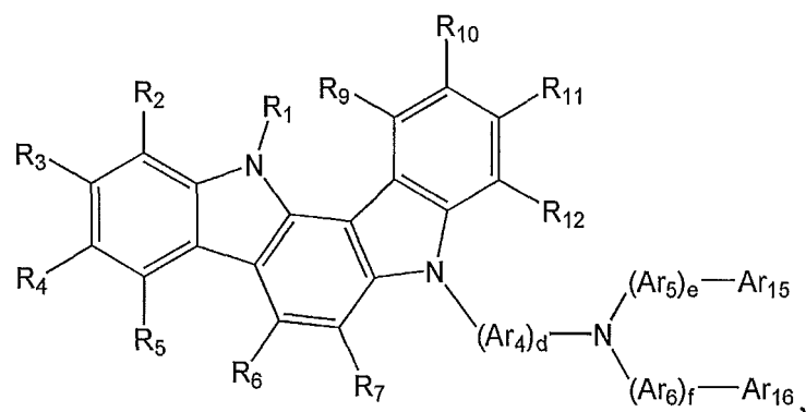
Formula 3e
