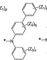
Formula 6E
