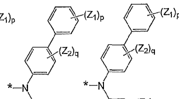
Formula 6E
