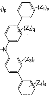
Formula 6F
