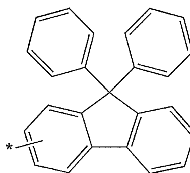
Formula 5E
