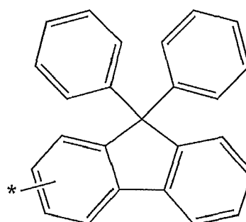
Formula 5E
