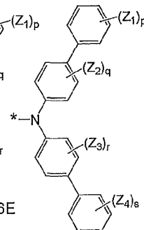
Formula 6F
