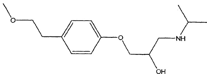
metoprolol
