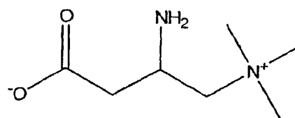
aminocarnitine
