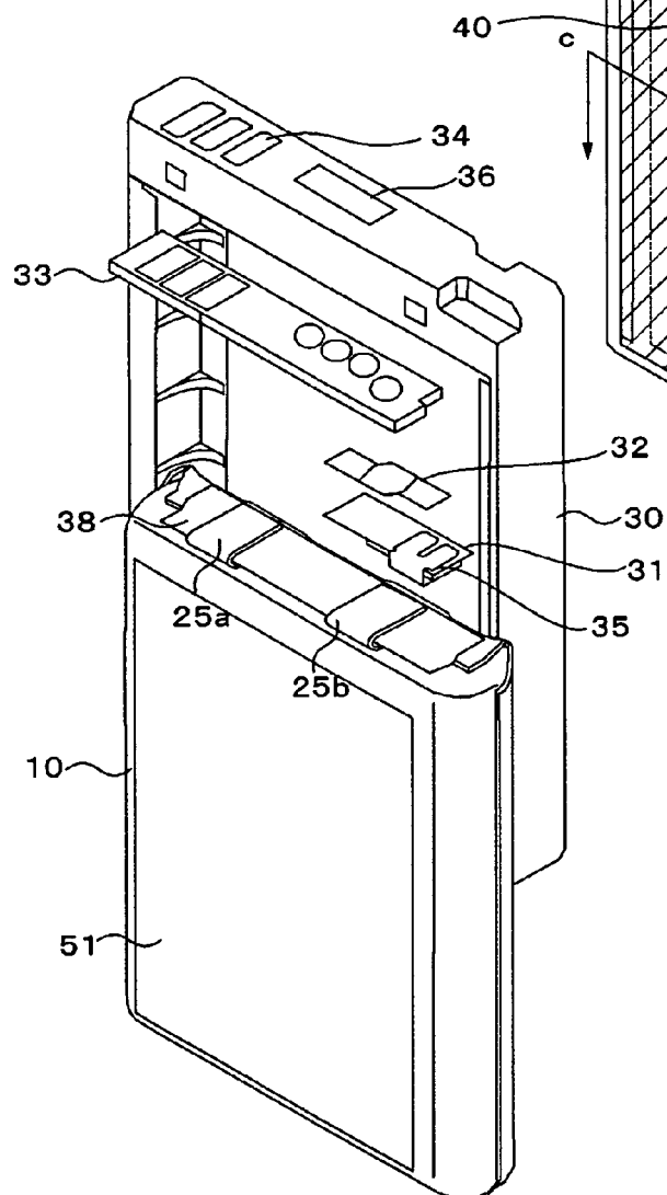
FIG. 7A
