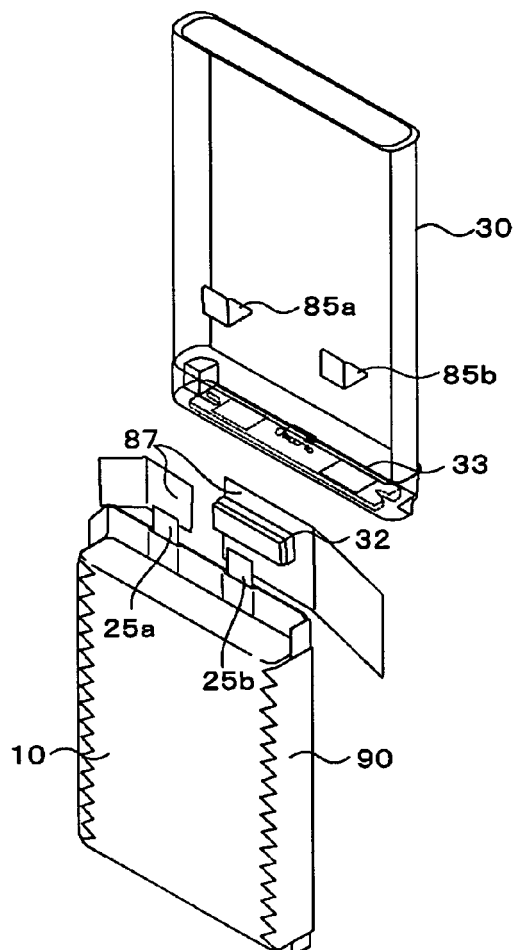
FIG. 13A
