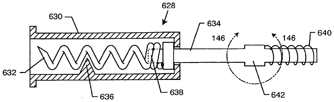
FIG. 145 PRIOR ART
