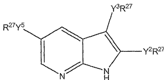
Formula Ir
