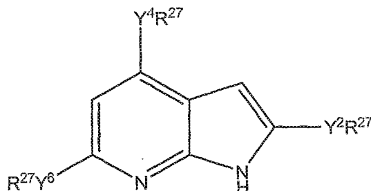
Formula Iu
