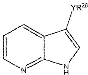
Formula Io
