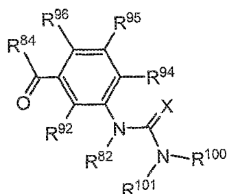
Formula VIIb
