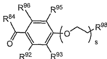
Formula Va
