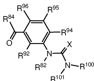
Formula VIIb
