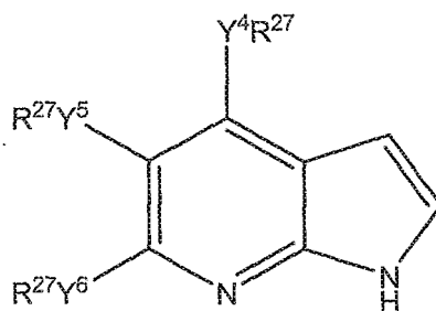
Formula Iz
