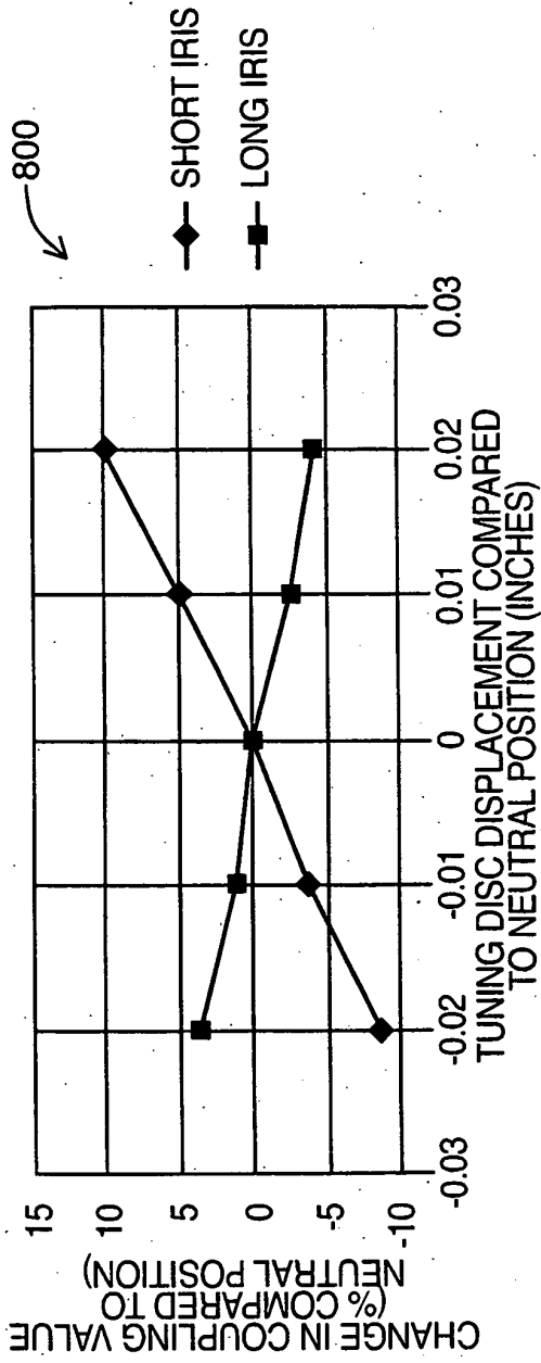
FIG. 8A
