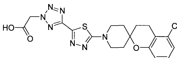
5-[5-(5-Chloro-3,4-dihydro-1' H -spiro[chromene-2,4'-piperidin]-1'-yl)-1,3,4-thiadiazol-2-yl]-2 H -tetrazol-2-yl]acetic acid
