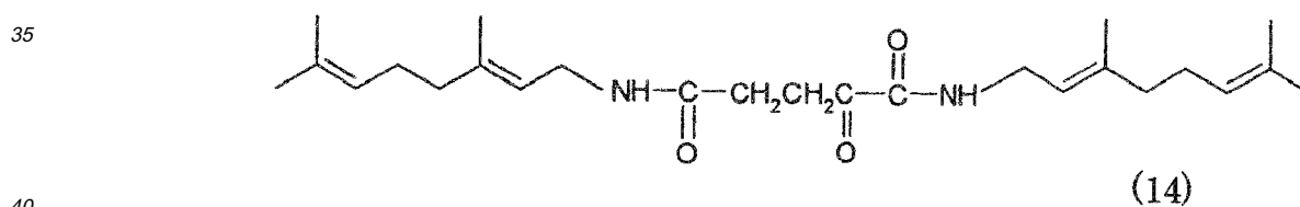
N-geranylpyruvamide
