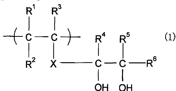
[Chem. 6]
